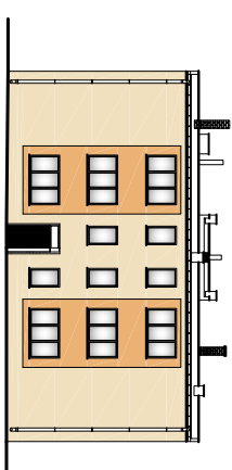
ELEWACJA PÓŁDNIOWA 1:100
