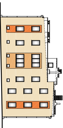
ELEWACJA ZACHODNIA 1:100
