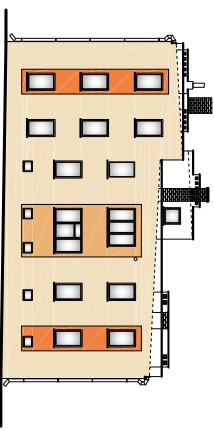
ELEWACJA WSCHODNIA 1:100
